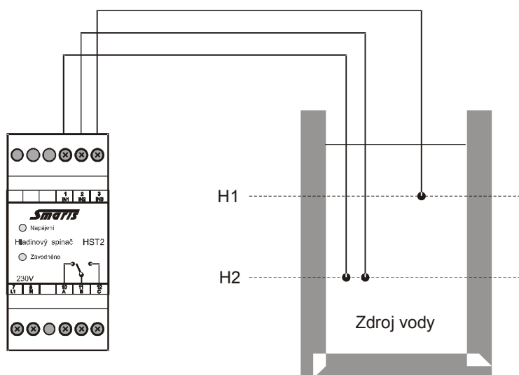
Zapojení vodivostních sond
